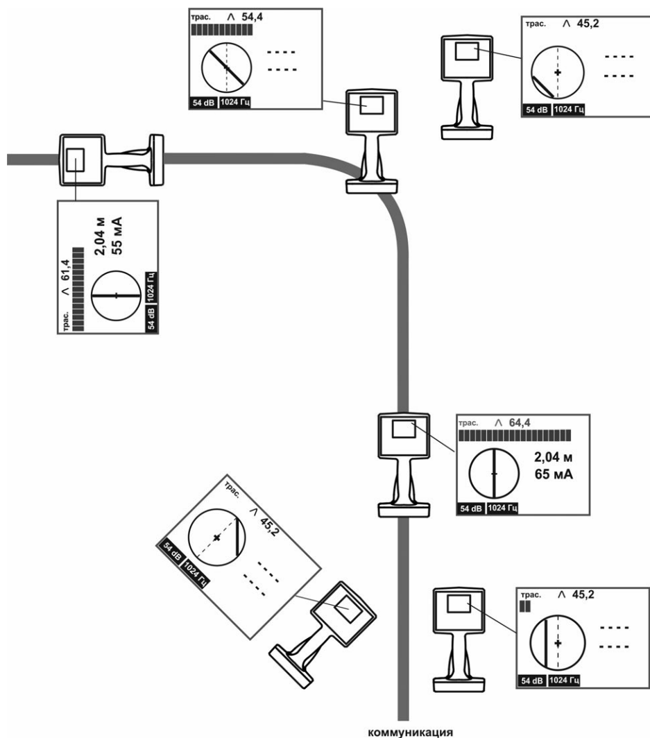
Рисунок 4.2.3 – Поиск с включенной функцией «КОМПАС»
