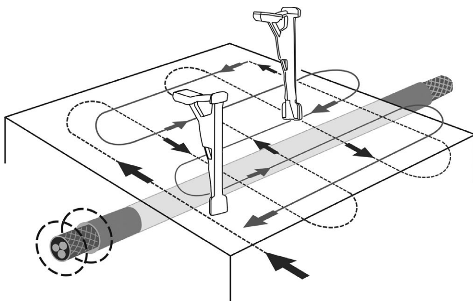
Рисунок 4.4.1 – Обследование участков местности без генератора
