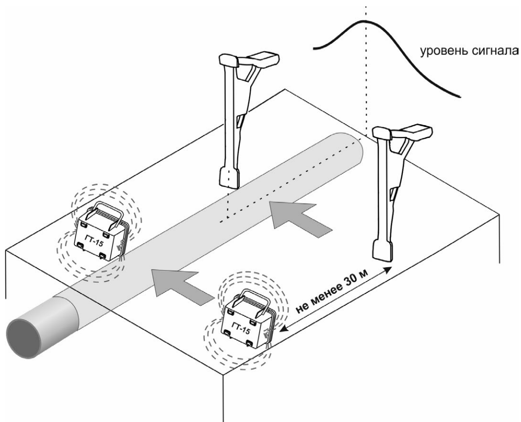
Рисунок 4.4.2.2 – Обследование участков местности с помощью ГТ-15
