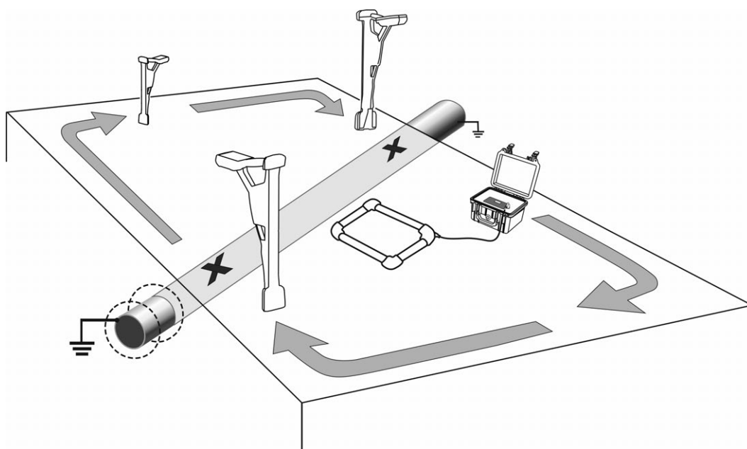
Рисунок 4.4.2.1 – Обследование участков местности с использованием рамки РП-02
