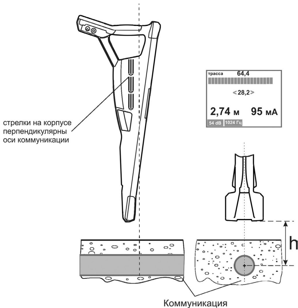
Рисунок 4.3 – Показания глубины залегания и тока
